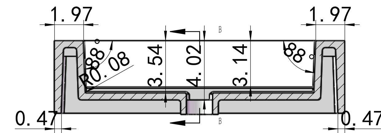
剖面 A-A 比例 1 : 4
