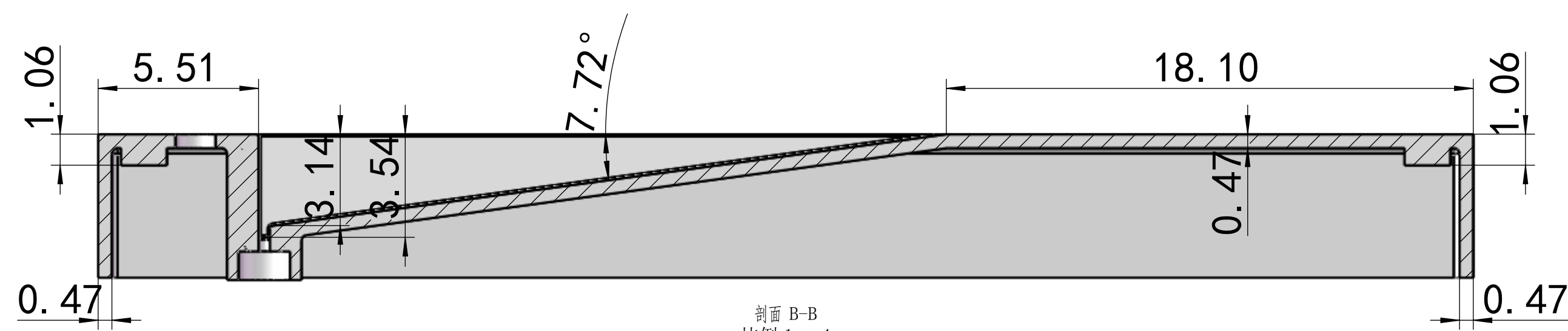
剖面 B-B 比例 1 : 4
