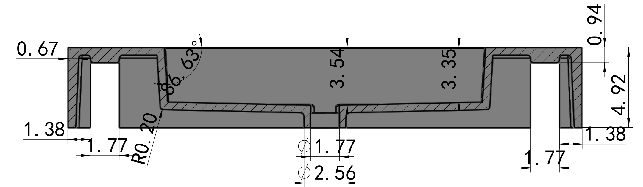
B-B 1 : 3.5
