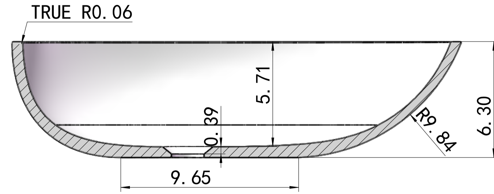
A-A 1:3
