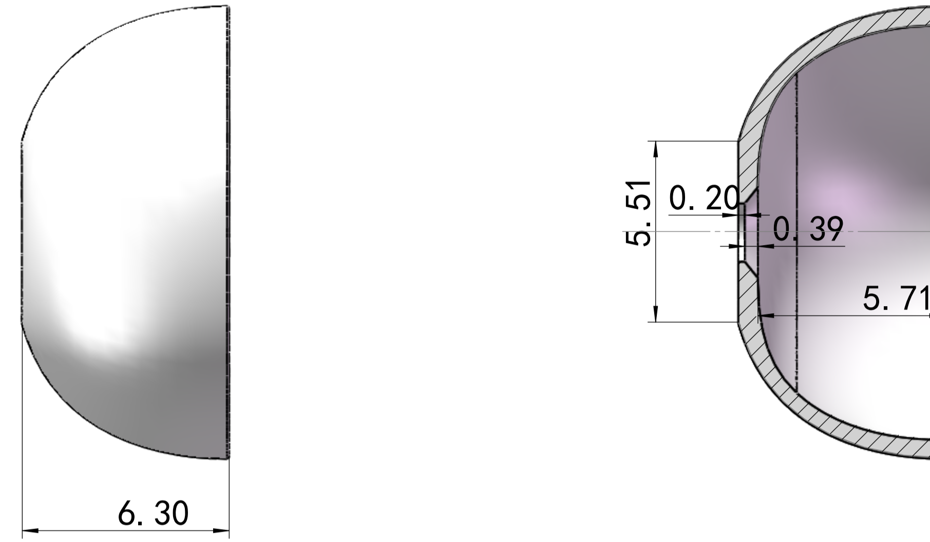
B-B 1:3
